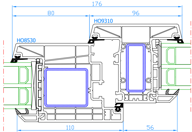
DPB-82 Setzpfosten Setzpfosten: HO9310 breiter Flügel: HO8530
