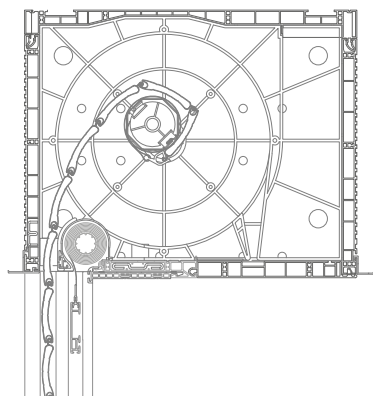
AUFSATZSYSTEM DK-RNB integriertes Insektenschutzgitter
