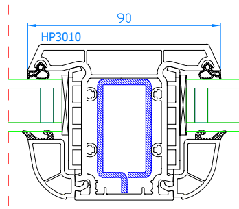
DPB-73 Setzpfosten Setzpfosten: HP3010
