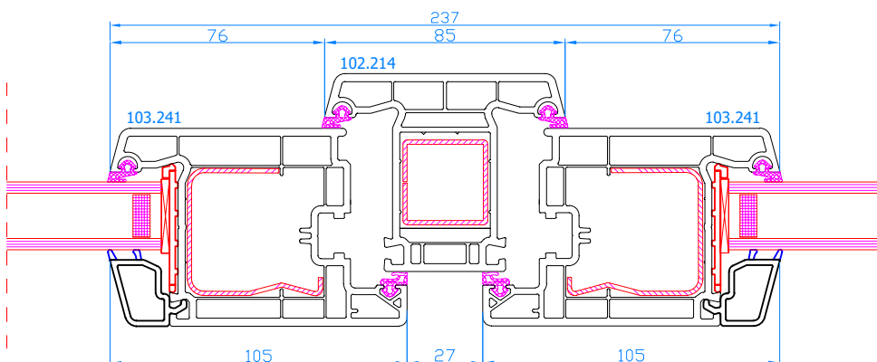
DPP-70 Setzpfosten Setzpfosten: 102.214 breiter Flügel: 103.241
