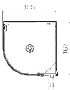
DK-RZP Kasten 165
