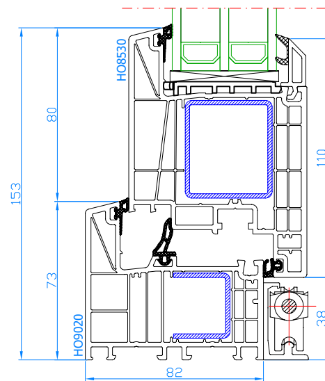
DPB-82 Parallell-Schiebe-Kipp-Tür >2,2 m 2 Rahmen: HO9020 breiter Flügel: HO8530
