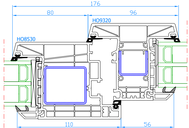
DPB-82 Setzposten Setzposten: HO9320 breiter Flügel: HO8530
