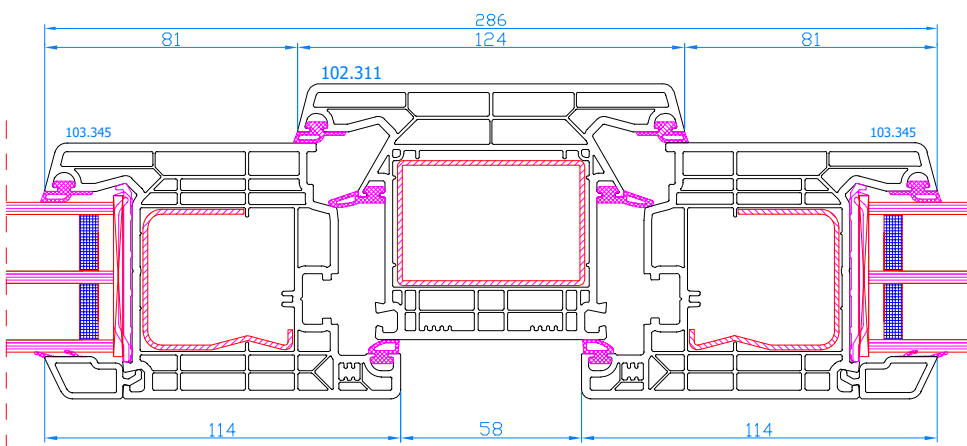
DPQ-82 Setzpfosten Setzpfosten: 102.311 breiter Flügel: 103.345
