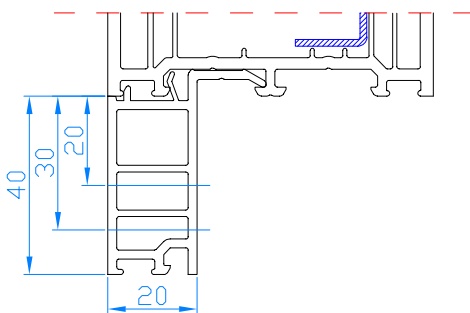
Fensterbankanschlußprofil 40x20
