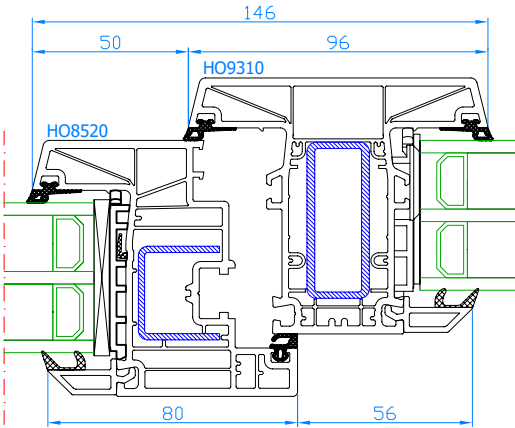
DPB-82 Setzpfosten Setzpfosten: HO9310 Flügel: HO8520
