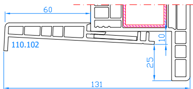
Fensterbankanschlußprofil für DPP-70 R35 Code: 110.102
