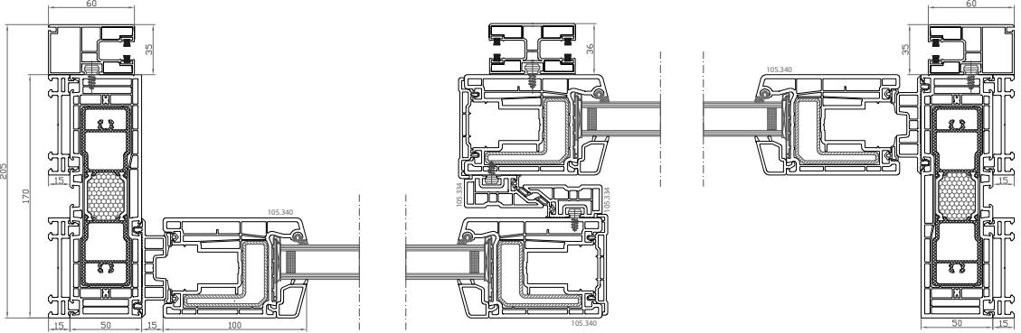
DPP-70 HST Aufsatzrollladen: DK-RNB Draufsicht
