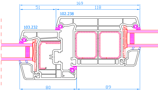
DPP-70 Setzpfosten Setzpfosten: 102.238 Flügel: 103.232
