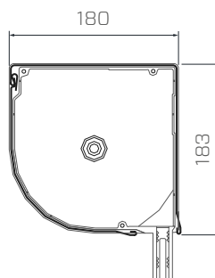
DK-RZP Kasten 180
