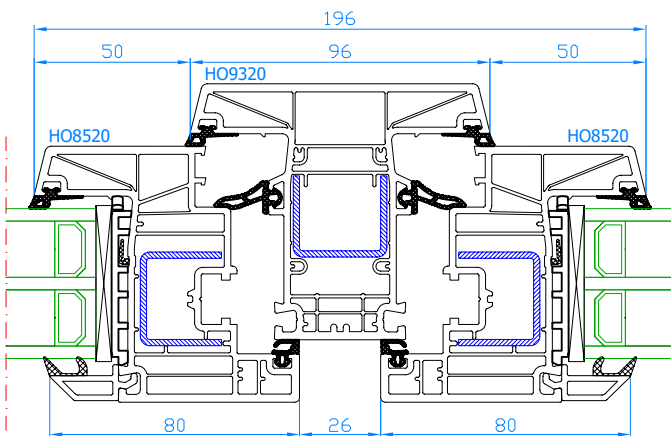
DPB-82 Setzposten Setzposten: HO9320 Flügel: HO8520
