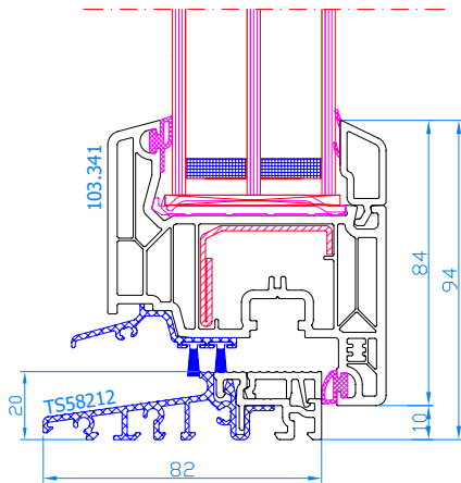
DPQ-82 Balkontür mit niedriger ALU-Schwelle nach innen öffnend ALU-Schwelle: TS58212 Flügel: 103.341
