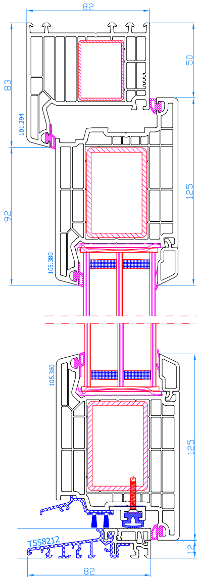
DPQ-82 Eingangstür mit niedriger ALU-Schwelle nach innen öffnend ALU-Schwelle: TS58212 Rahmen: 101.294 Flügel: 105.380
