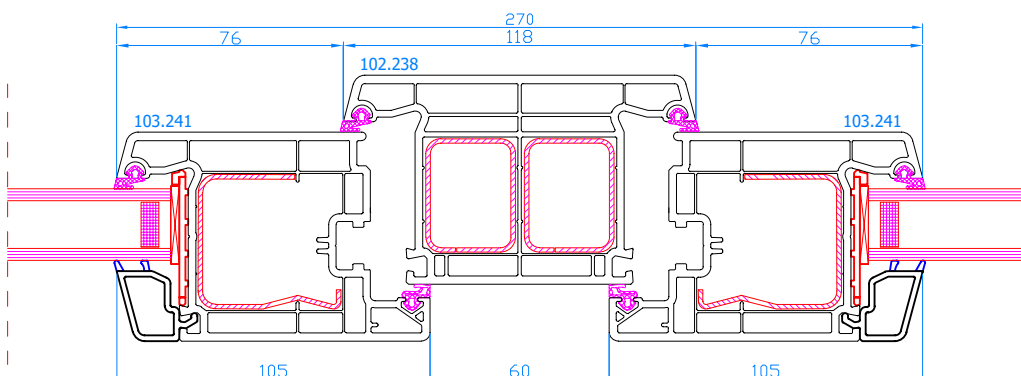
DPP-70 Setzpfosten Setzpfosten: 102.238 breiter Flügel: 103.241
