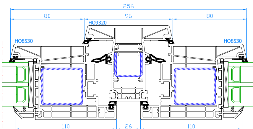
DPB-82 Setzposten Setzposten: HO9320 breiter Flügel: HO8530
