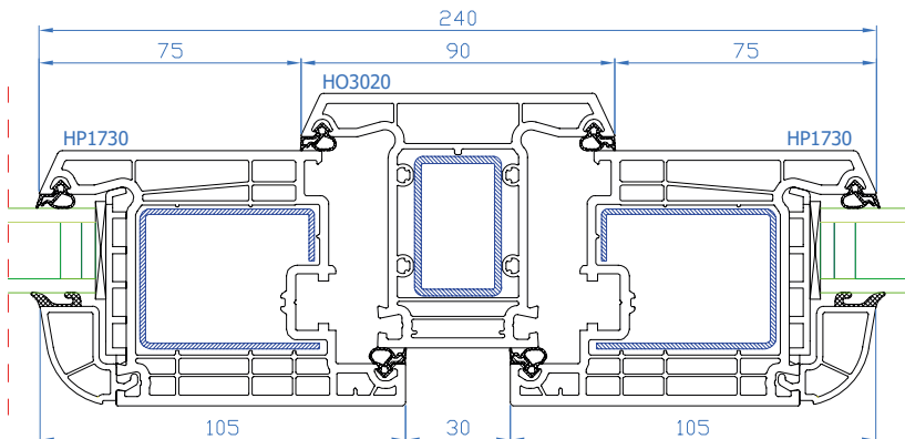
DPB-73 Setzpfosten Setzpfosten: HO3020 breiter Flügel: HP1730
