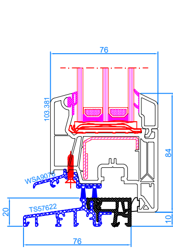
DPQ-76 Balkontür mit niedriger ALU-Schwelle nach innen öffnend ALU-Schwelle: TS57622 Flügel: 103.381
