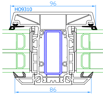
DPB-82 Setzpfosten Setzpfosten: HO9310
