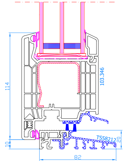
DPQ-82 Balkontür mit niedriger ALU-Schwelle nach außen öffnend ALU-Schwelle: TS58212 breiter Flügel: 103.346
