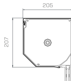
DK-RZS Kasten 205
