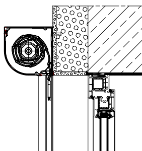
DK-RZP vorne an der Wand montiert
