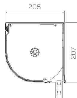
DK-RZP Kasten 205
