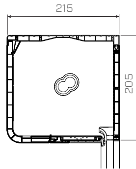
DK-RNC Kasten 205
