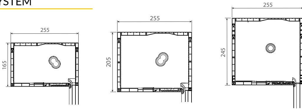
DK-RNB Kasten 165
