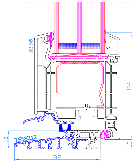
DPQ-82 Balkontür mit niedriger ALU-Schwelle nach innen öffnend ALU-Schwelle: TS58212 breiter Flügel: 103.345
