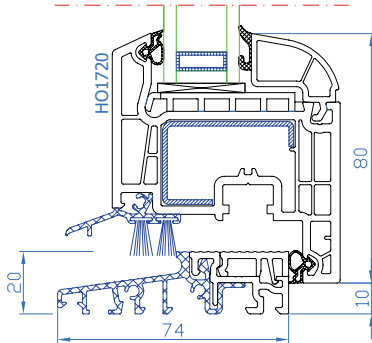
DPB-73 Balkontür mit niedriger ALU-Schwelle ALU-Schwelle: TS57412 Flügel: HO1720
