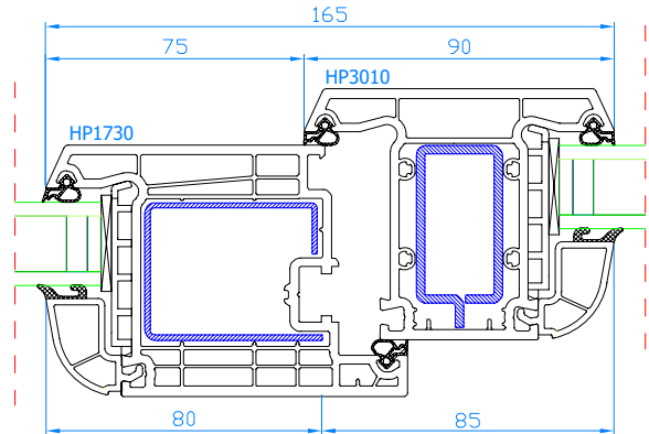
DPB-73 Setzpfosten Setzpfosten: HP3010 breiter Flügel: HP1730
