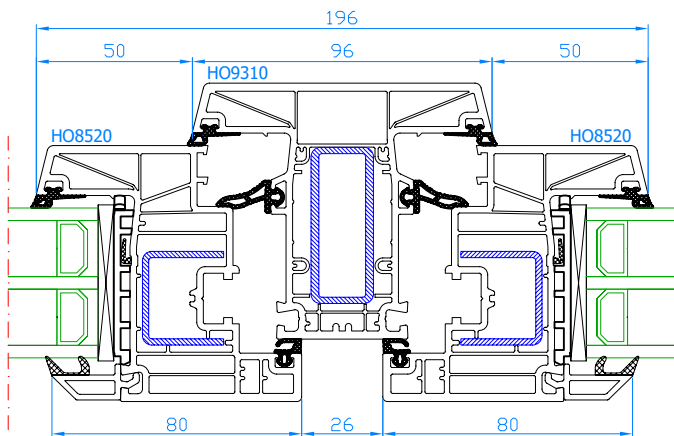
DPB-82 Setzpfosten Setzpfosten: HO9310 Flügel: HO8520
