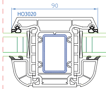
DPB-73 Setzpfosten Setzpfosten: HO3020
