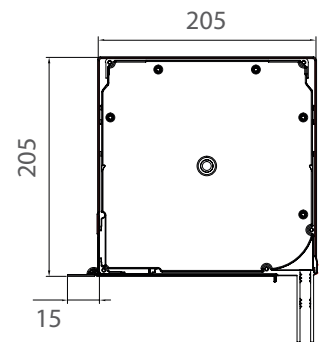
DK-RSP Kasten 205
