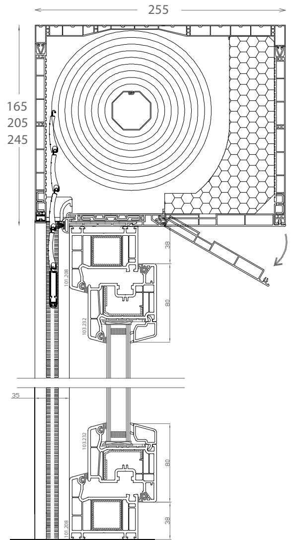
DPP-70 Aufsatzrollladen: DK-RNB Querschnitt
