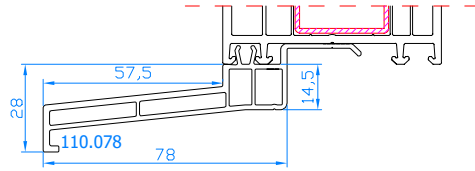
Fensterbankanschlußprofil 28x78 Code: 110.078
