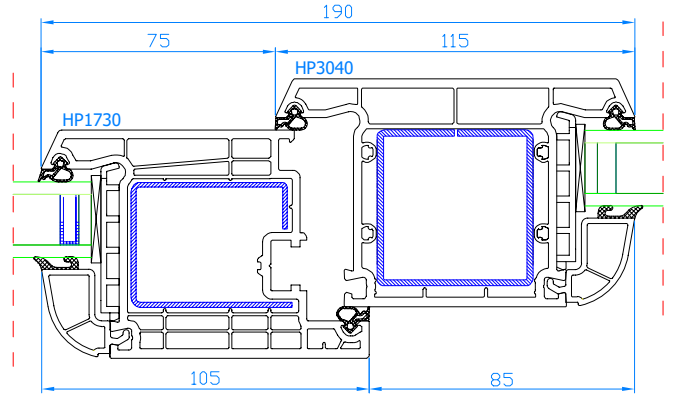
DPB-73 Setzpfosten Setzpfosten: HP3040 breiter Flügel: HP1730
