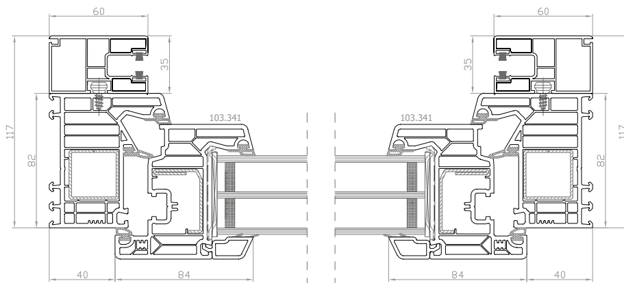
DPQ-82 Draufsicht
