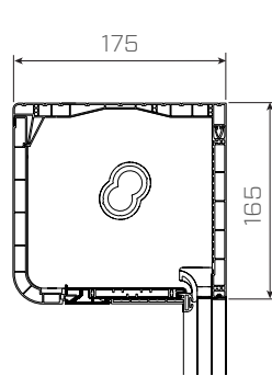
DK-RNC Kasten 165
