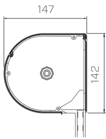
DK-RZO Kasten 137
