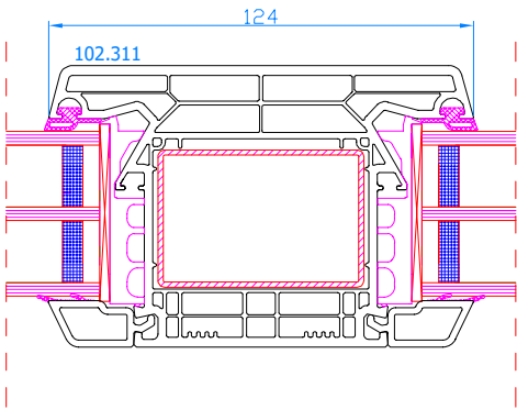
DPQ-82 Setzpfosten Setzpfosten: 102.311
