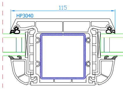
DPB-73 Setzpfosten Setzpfosten: HP3040
