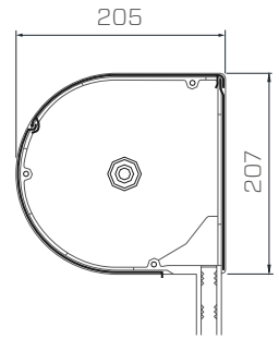
DK-RZO Kasten 205
