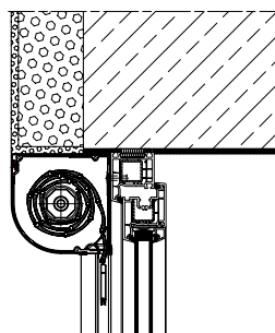
DK-RZP in der Nische montiert
