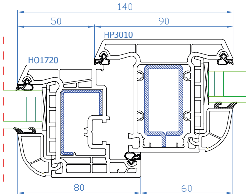
DPB-73 Setzpfosten Setzpfosten: HP3010 Flügel: HO1720
