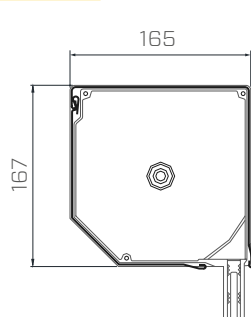
DK-RZS Kasten 165
