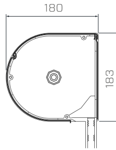
DK-RZO Kasten 180
