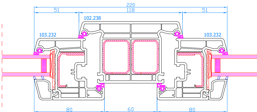
DPP-70 Setzpfosten Setzpfosten: 102.238 Flügel: 103.232
