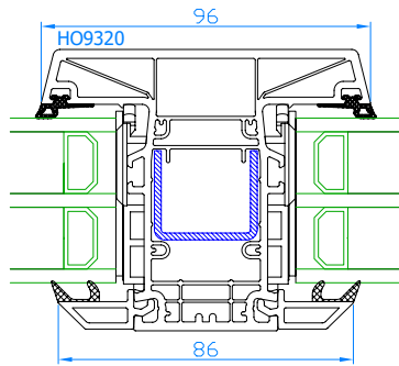
DPB-82 Setzposten Setzposten: HO9320
