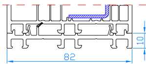
Verbreiterungen 10mm Code: NP8200 für DPB-82
