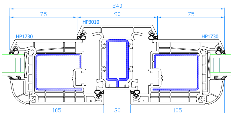
DPB-73 Setzpfosten Setzpfosten: HP3010 breiter Flügel: HP1730
