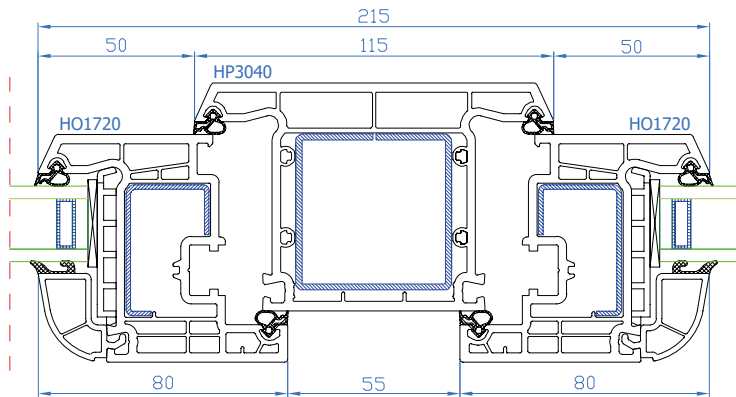
DPB-73 Setzpfosten Setzpfosten: HP3040 Flügel: HO1720
