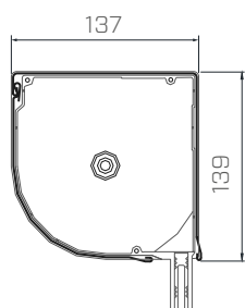
DK-RZP Kasten 137
