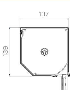
DK-RZS Kasten 137
