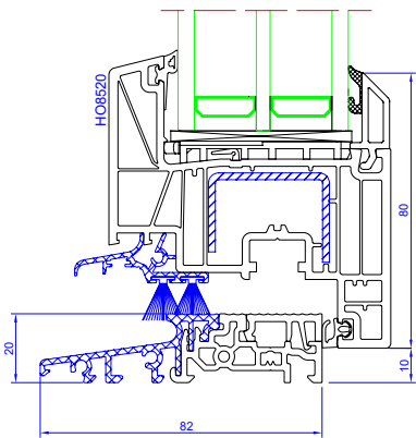
DPB-82 Balkontür mit niedriger ALU-Schwelle ALU-Schwelle: TS88210 Flügel: HPO1820
