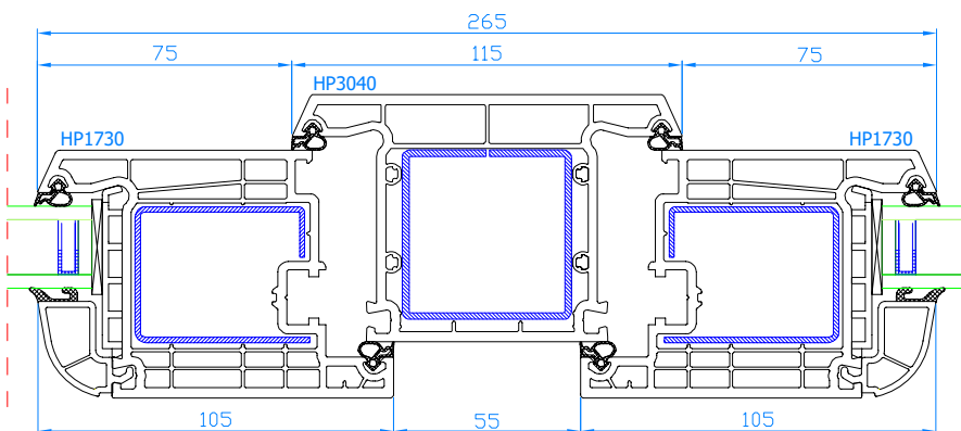
DPB-73 Setzpfosten Setzpfosten: HP3040 breiter Flügel: HP1730
