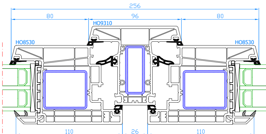
DPB-82 Setzpfosten Setzpfosten: HO9310 breiter Flügel: HO8530
